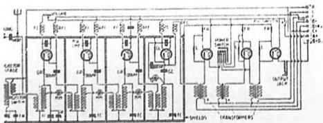
Diagrama completo de la instalación del receptor de siete válvulas. Los rectángulos de líneas sombreadas representan los blindajes.
