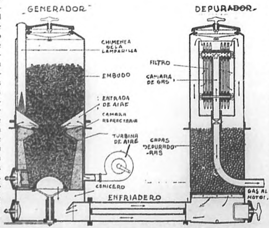
Detalles de la instalación Panhard para la alimentación de motores ligeros.
